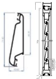
BEWEGLICH Regelung des Licht- und Lüftflusses
